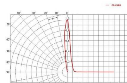
Исполнение «К15»
