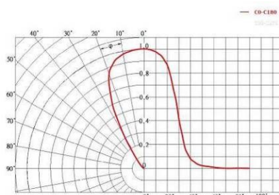
Исполнение «Г60»
