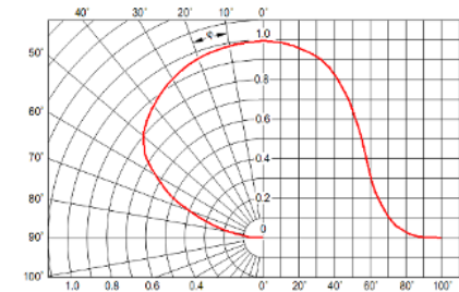
Исполнение «Д»
